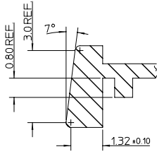
A-A SCALE 10:1
